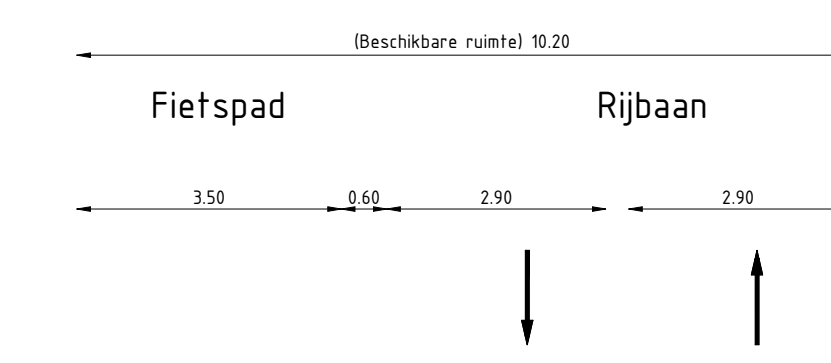
Principe dwarsprofiel B-B VRI kruispunt Schaal 1:100
