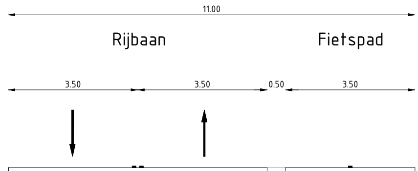
Principe dwarsprofiel A-A Schaal 1:100
