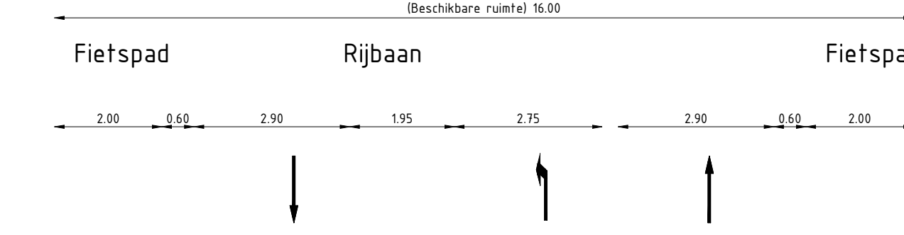
Principe dwarsprofiel A-A VRI kruispunt Schaal 1:100
