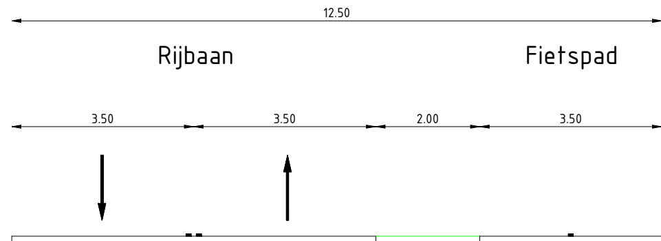
Principe dwarsprofiel A-A Schaal 1:100
