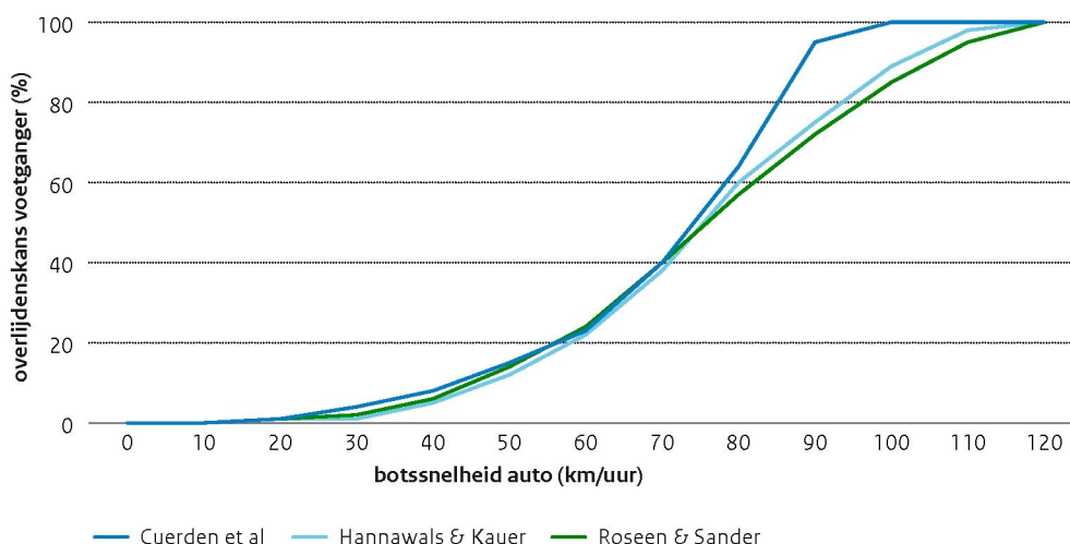
Figuur 7: Overlijdenskans in relatie tot snelheid (bron: SWOV - Snelheid en verkeersmanagement (2016))
