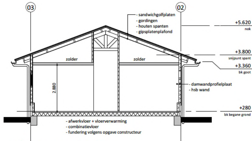
doorsnede A
