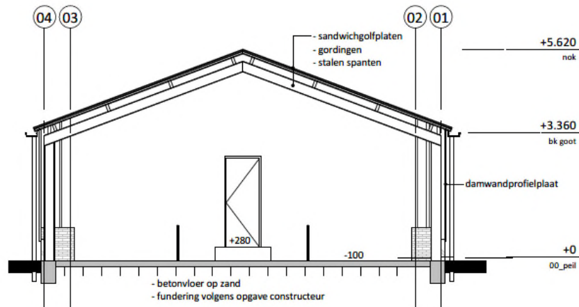
doorsnede B
