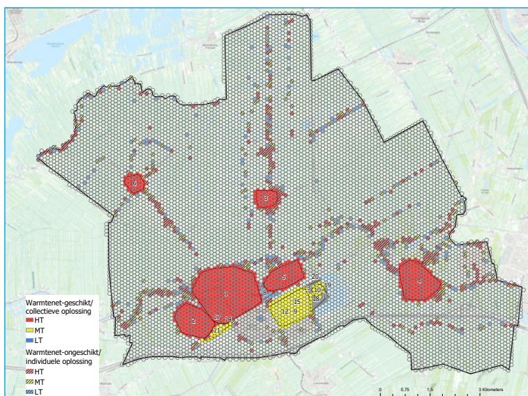
Figuur 8: Benodigde verwarmingstemperatuur voor isolatie. HT (hoge temperatuur) betekent verwarming op meer dan 70°C. MT (midden temperatuur) betekent verwarming op 50-70°C en LT (lage temperatuur) betekent verwarming op lager dan 50°C.
