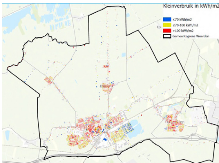
Figuur 6: Huidig, geüniformeerd warmteverbruik van met name woningen per m² vloeroppervlak.
