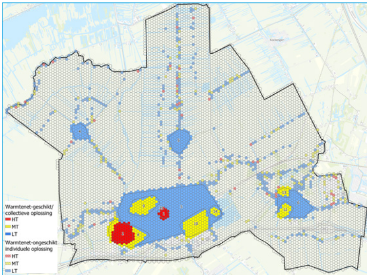
Figuur 9: Benodigde verwarmingstemperatuur na isolatie. HT (hoge temperatuur) betekent verwarming op meer dan 70°C. MT (midden temperatuur) betekent verwarming op 50-70°C en LT (lage temperatuur) betekent verwarming op lager dan 50°C.
