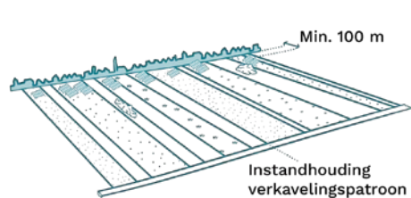
Ontwerpprincipe 4: kleinschalige zonnevelden op kavels achter de bebouwingslinten
