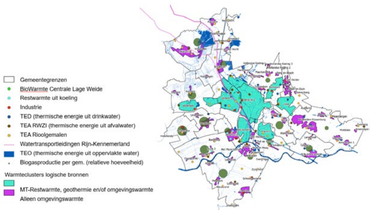
Figuur 4.5. Een overzicht van warmtevraagclusters met bovengemeentelijke potentie en warmtevraagclusters met lokale warmtebronnen.
