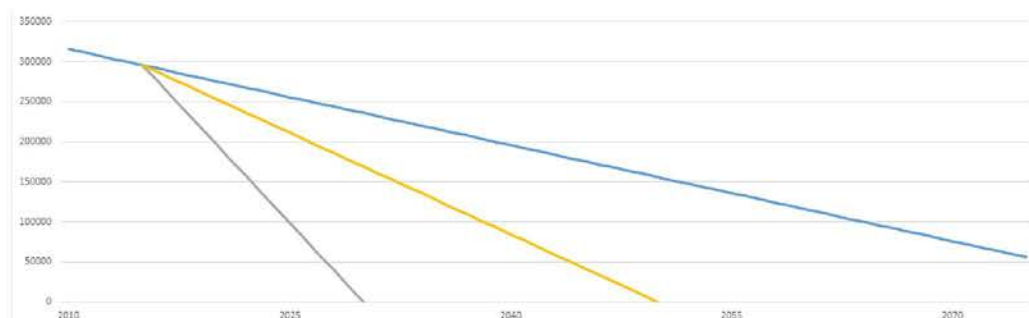
Figuur 6: CO 2 -uitstoot gemeente Woerden. Blauw: scenario "taak", geel: scenario "Tempo", grijs: scenario "Turbo".
