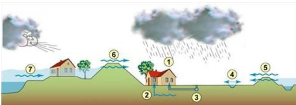
Figuur 2 Oorzaken van wateroverlast en overstroming (Klopstra, D. & M. Kok, 2009).
