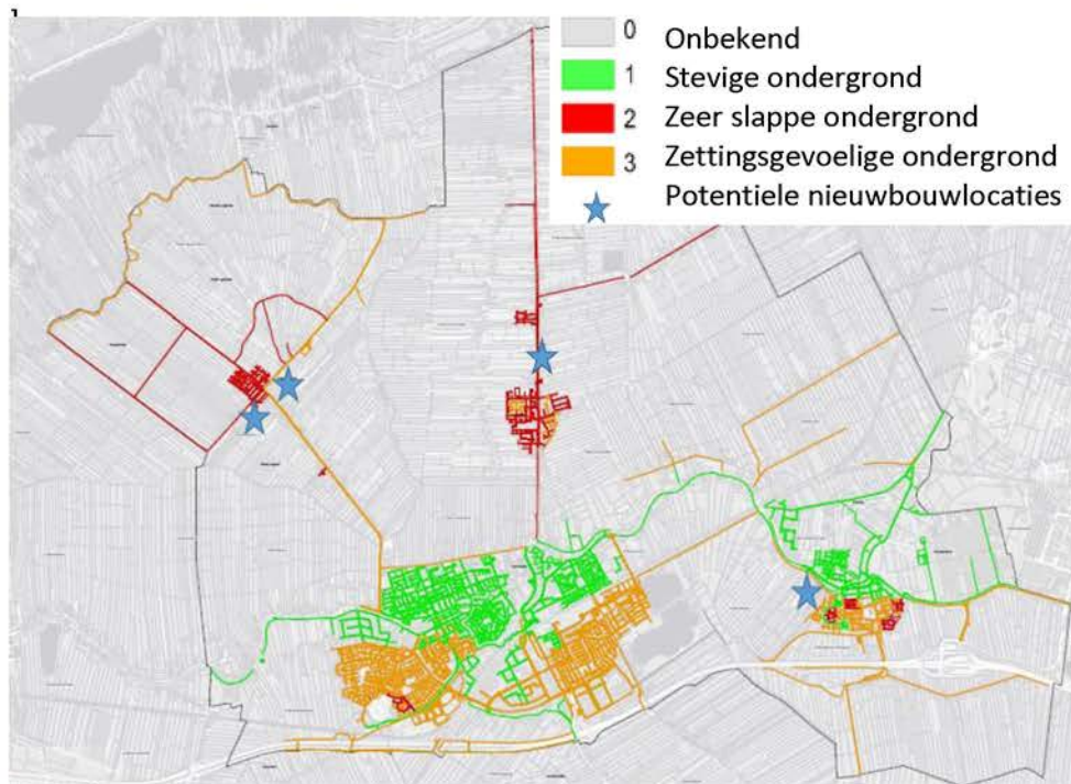
Figuur 2: Bodemcategorieën openbare ruimte op basis van data en expertise
