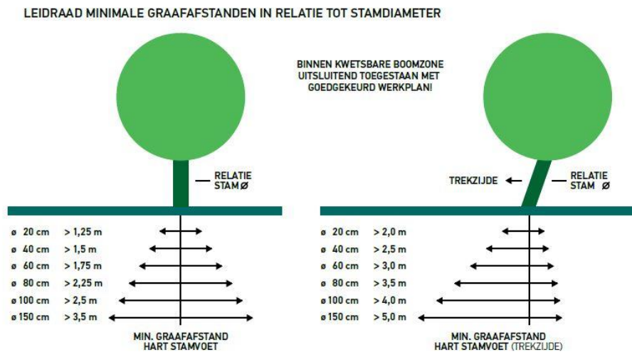
Afbeelding 2 Leidraad minimale graafafstand
