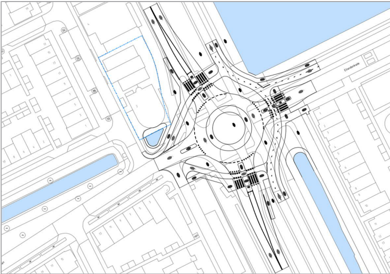
Figuur 20: variant 2B: enkelstrooksrotonde met fietsoversteken in één richting over de Steinhagenseweg
