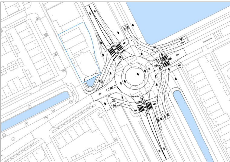
Figuur 2: 'overall' voorkeursvariant 2A: enkelstrooksrotonde met fietsoversteken in één richting over de Steinhagenseweg
